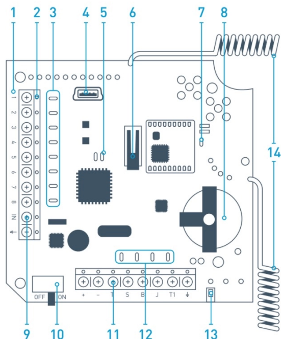
Рис. 1. Приемник беспроводных датчиков ocBridge Plus
