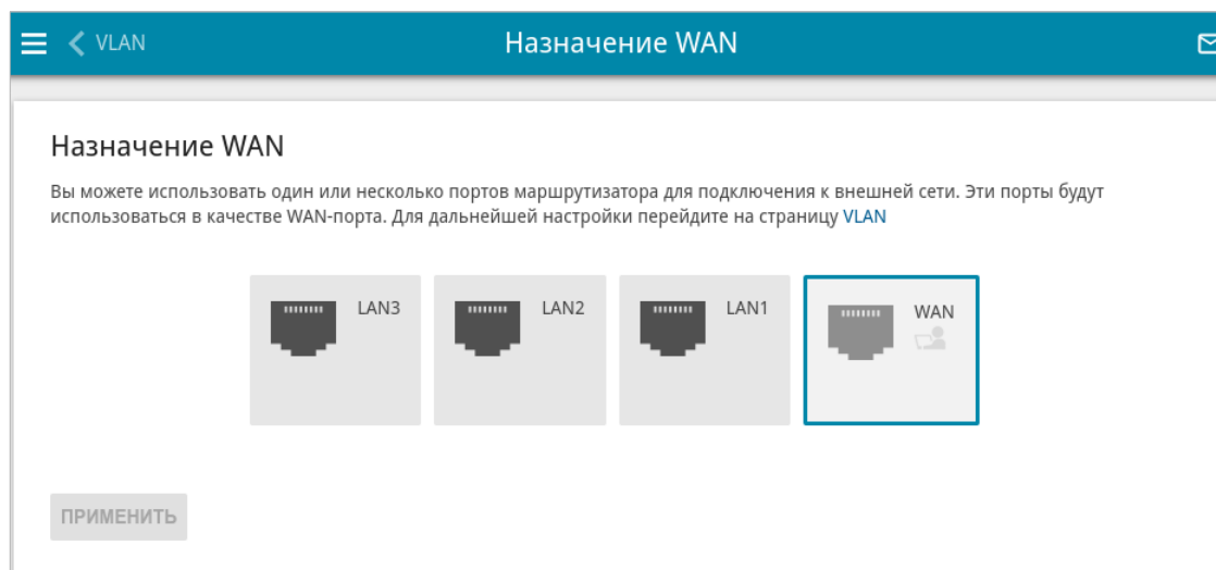
Рисунок 111. Страница Дополнительно / Назначение WAN .
