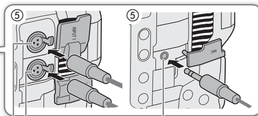
Разъем INPUT 2
