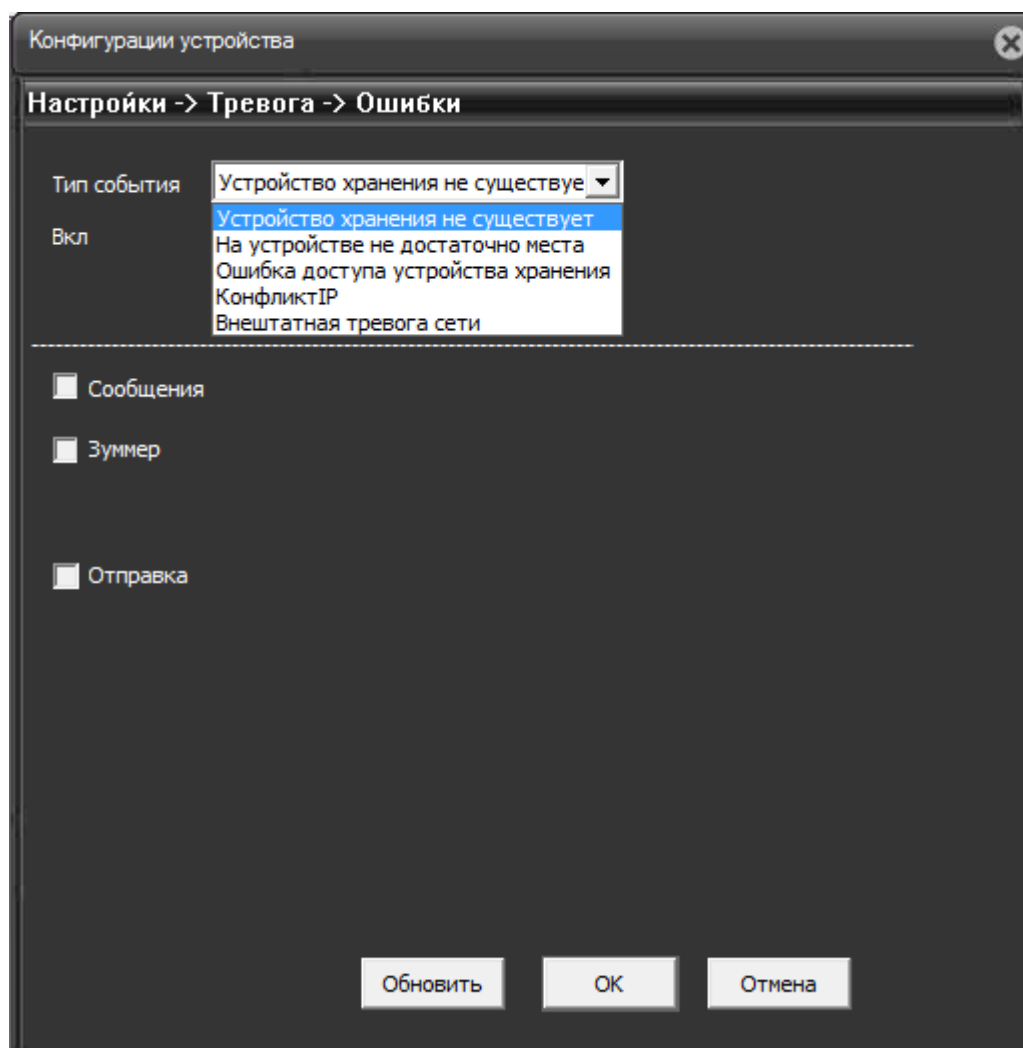
Рис. 8.4.4.1. Вкладка «Настройки-Тревога-Ошибки».
