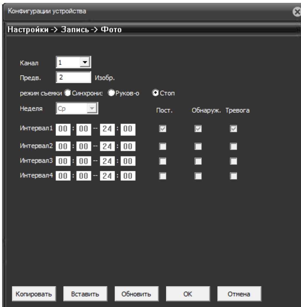
Рис. 8.3.2.1. Вкладка «Фото».
