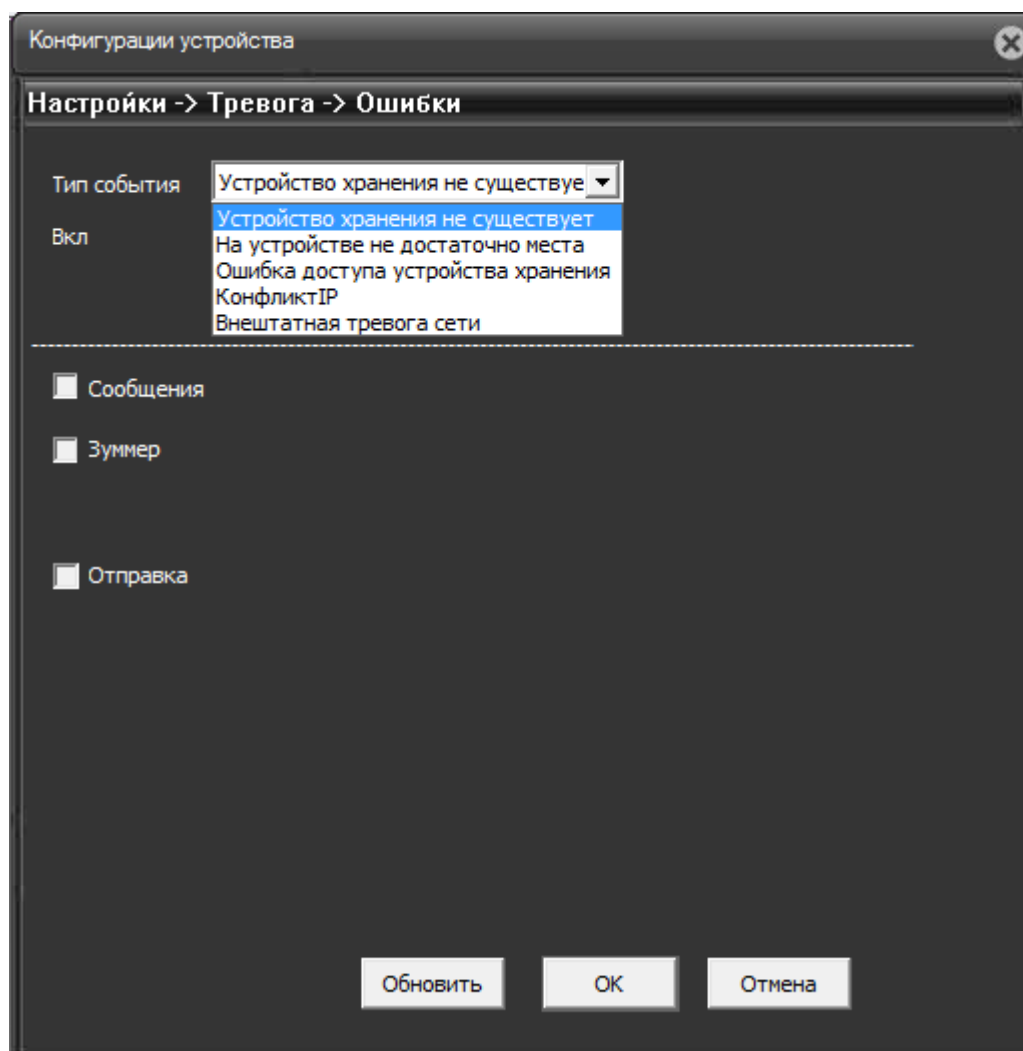
Рис. 8.4.4.1. Вкладка «Настройки-Тревога-Ошибки».
