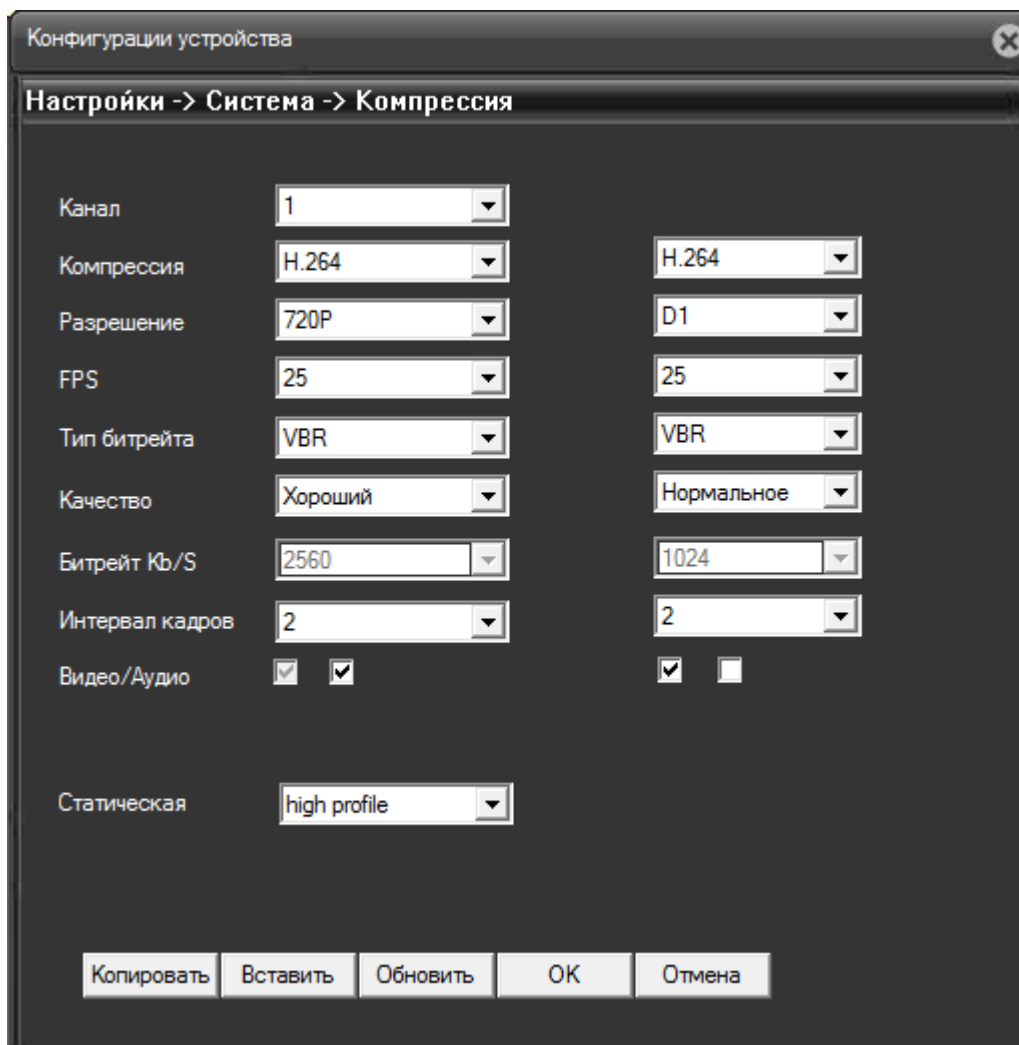
Рис. 8.5.2.1. Вкладка «Настройки-Система-Компрессия».
