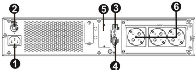
Schuko Type
