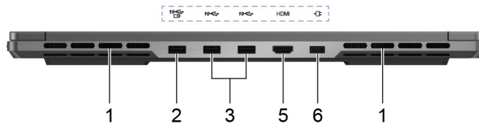
Малюнок 1. Вид ззаду— Legion Slim 7 16IRH8 і Lenovo Legion Slim 7 16IRH8 D2
