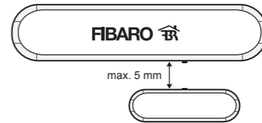
Схема 4 – Схема расположения Датчика и магнита
