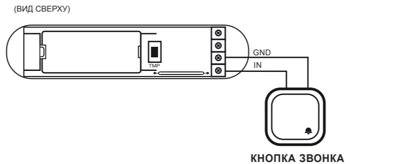
Схема 3 – Пример подключения моностабильного выключателя
