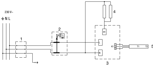
6 Сурет: Электрсхемасы
