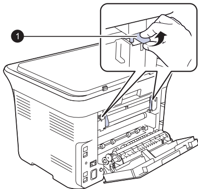
1 рычаг термофиксатора
