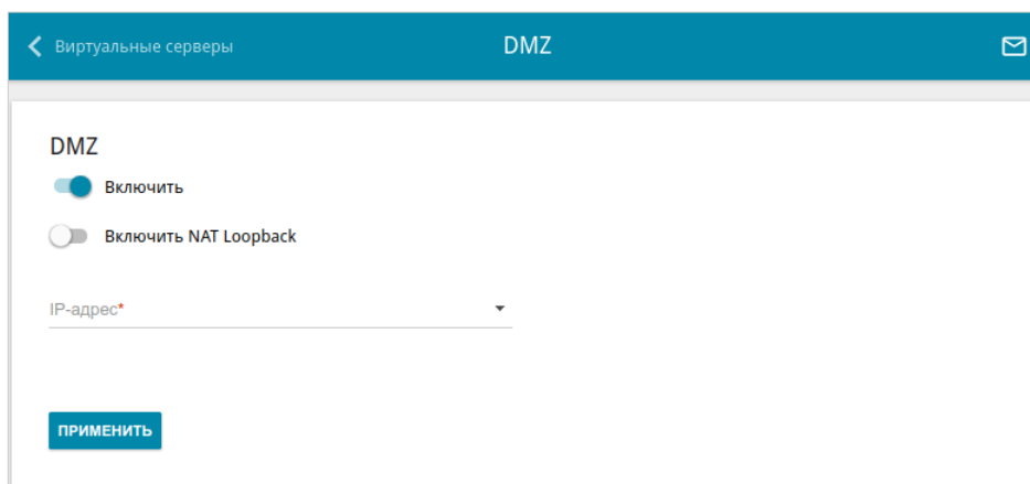
Рисунок 126. Страница Межсетевой экран / DMZ .
