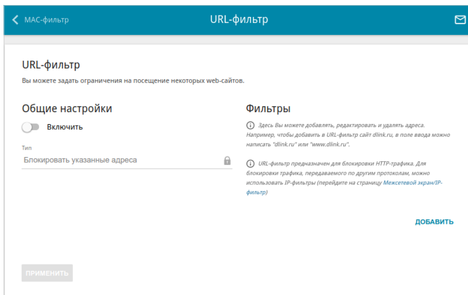
Рисунок 129. Страница Межсетевой экран / URL-фильтр .
