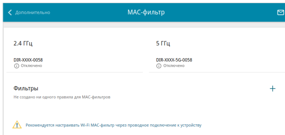
Рисунок 94. Страница для настройки MAC-фильтра для беспроводной сети.
