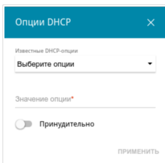
Рисунок 76. Окно для настройки опции DHCP.
