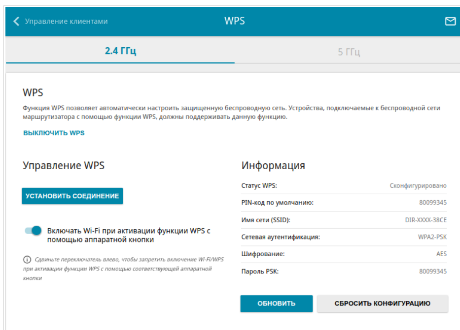
Рисунок 89. Страница для настройки функции WPS.
