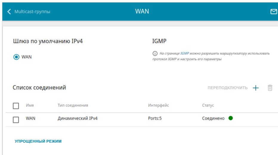
Рисунок 51. Страница Настройка соединений / WAN . Расширенный режим.
