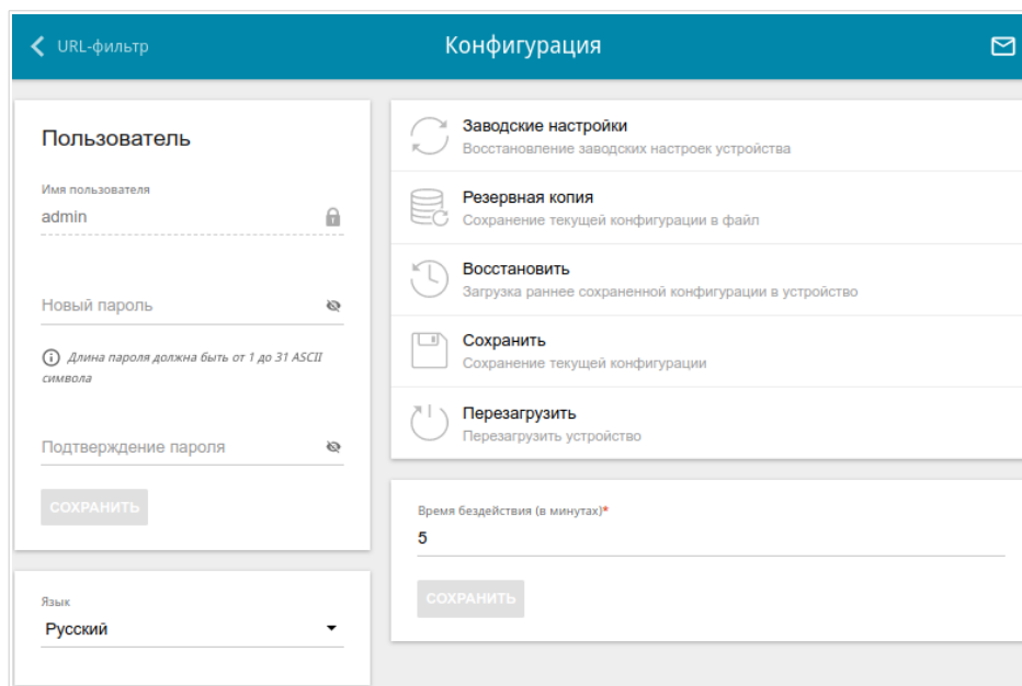
Рисунок 130. Страница Система / Конфигурация .
