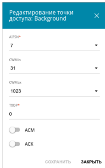
Рисунок 91. Окно для изменения параметров функции WMM.
