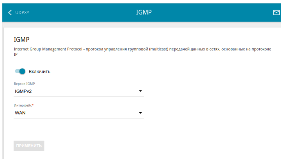
Рисунок 116. Страница Дополнительно / IGMP .
