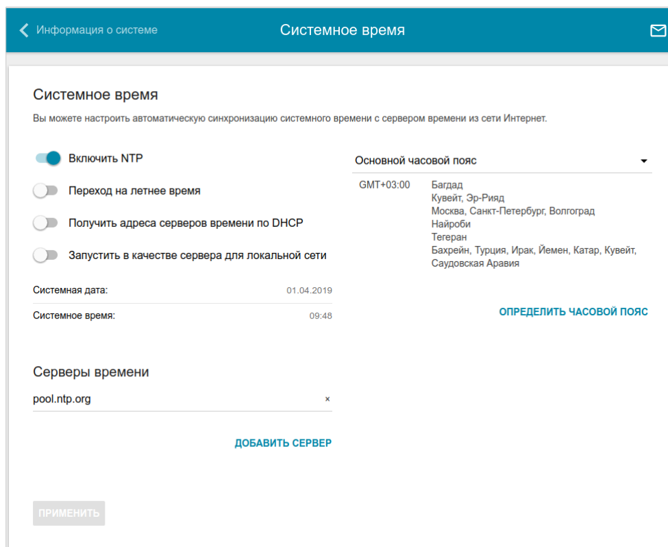
Рисунок 139. Страница Система / Системное время .
