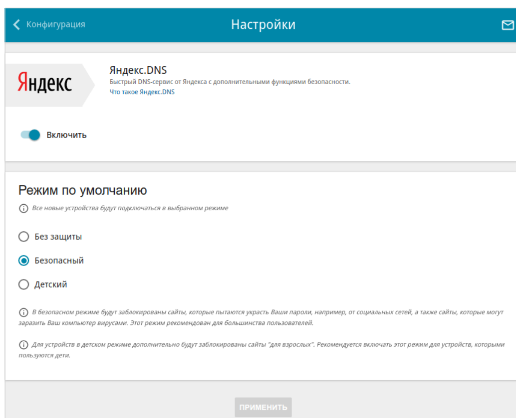
Рисунок 140. Страница Яндекс.DNS / Настройки .
