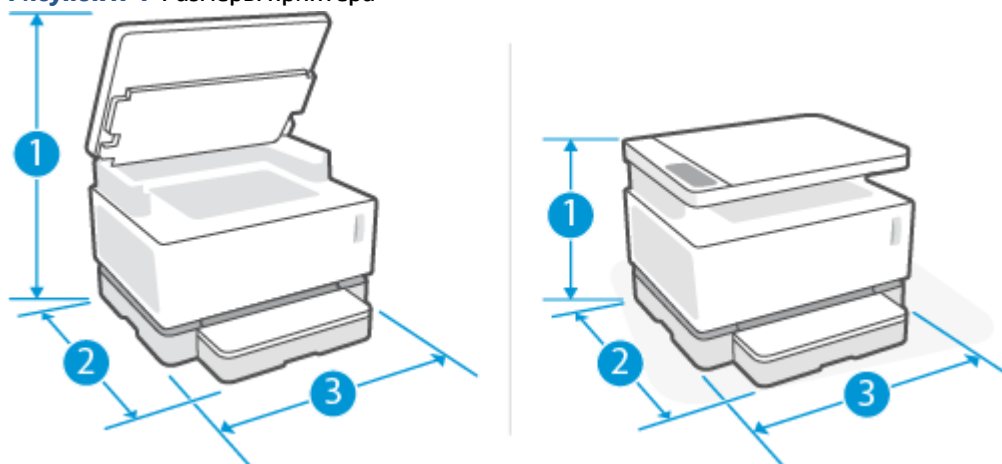
Рисунок А-1 Размеры принтера
