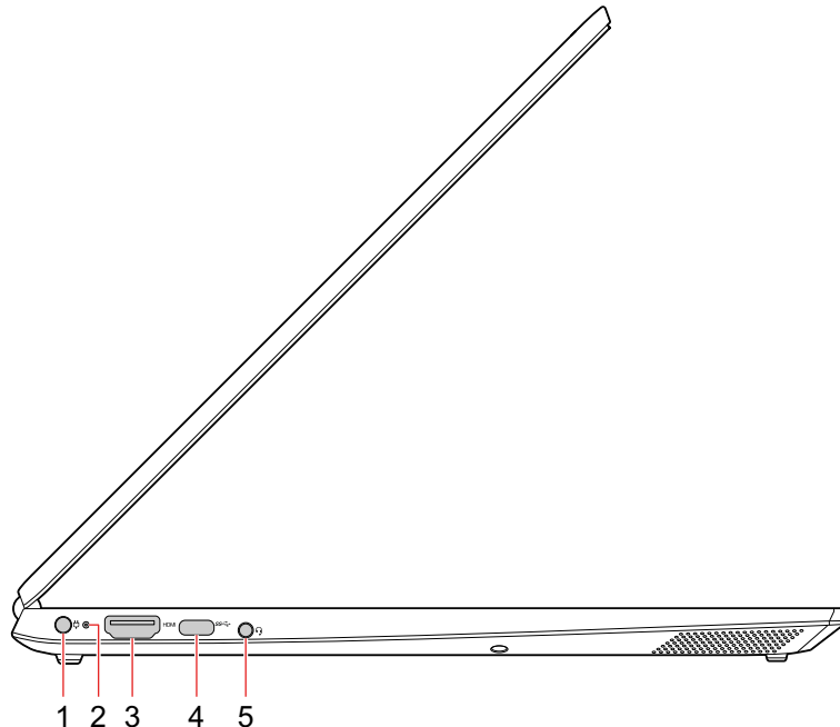
Рис. 5. Серия Lenovo IdeaPad S340-14/15 – вид слева
