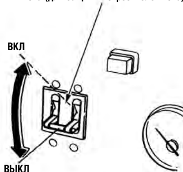
Предохранитель цепи переменного тока (для защиты потребителей тока)
