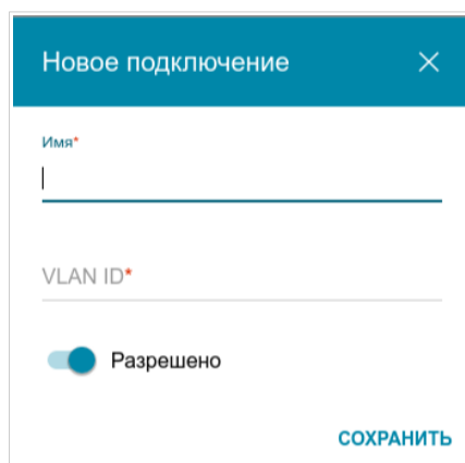
Рисунок 44. Добавление подключения.
