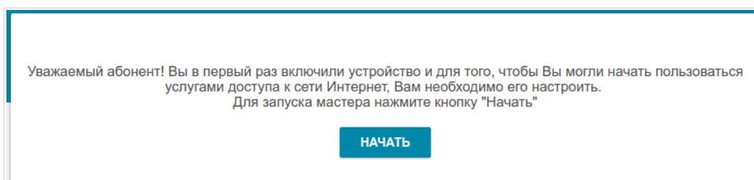
Рисунок 20. Запуск Мастера.
