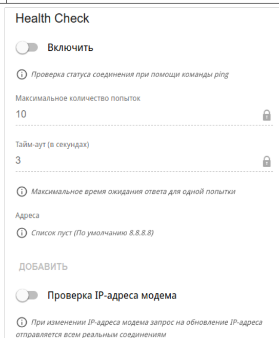
Рисунок 87. Страница добавления соединения типа Мобильный интернет . Раздел Health Check .
