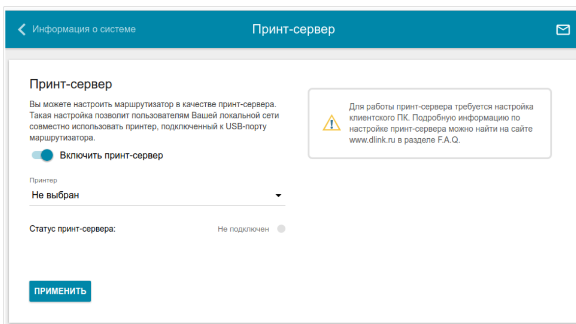
Рисунок 130. Страница Принт-сервер .
