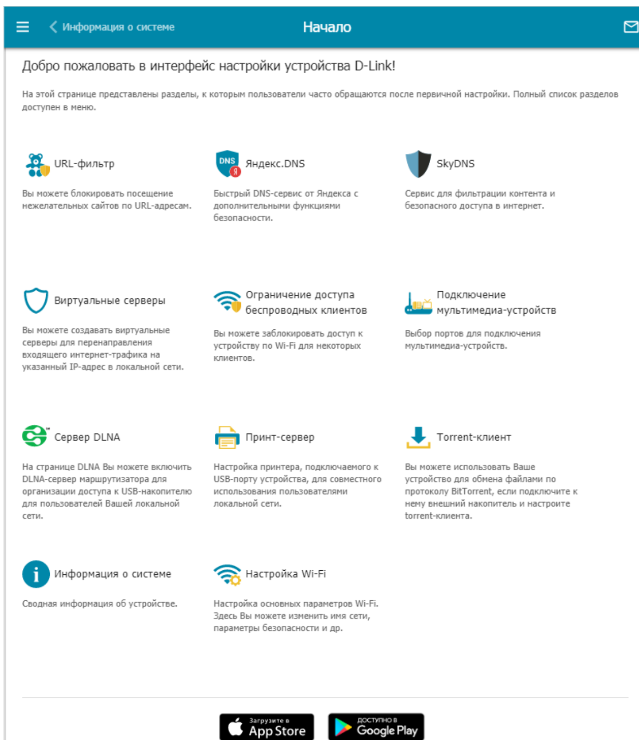
Рисунок 26. Страница Начало .
