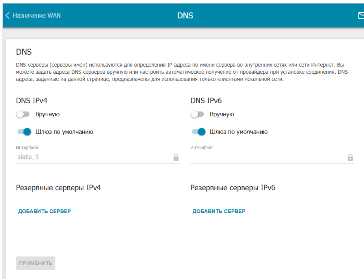
Рисунок 157. Страница Дополнительно / DNS .
