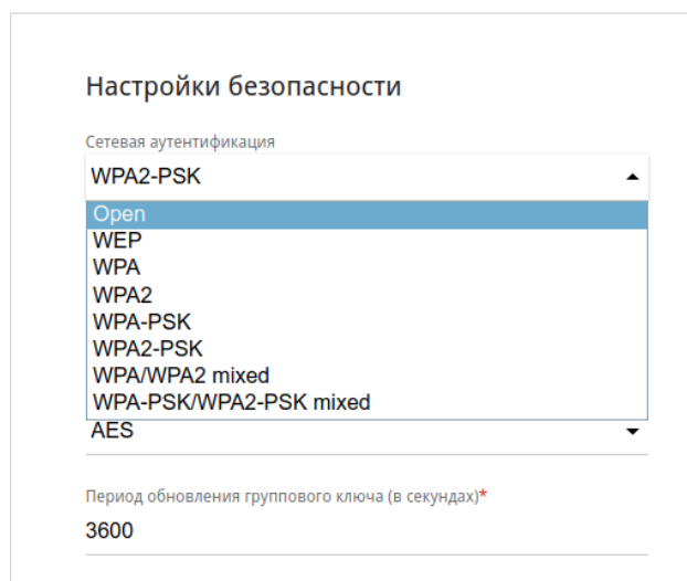
Рисунок 117. Типы аутентификации, поддерживаемые маршрутизатором.
